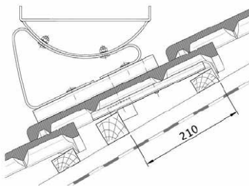
Schemat montażu strzemienia pod ławę kominiarską
